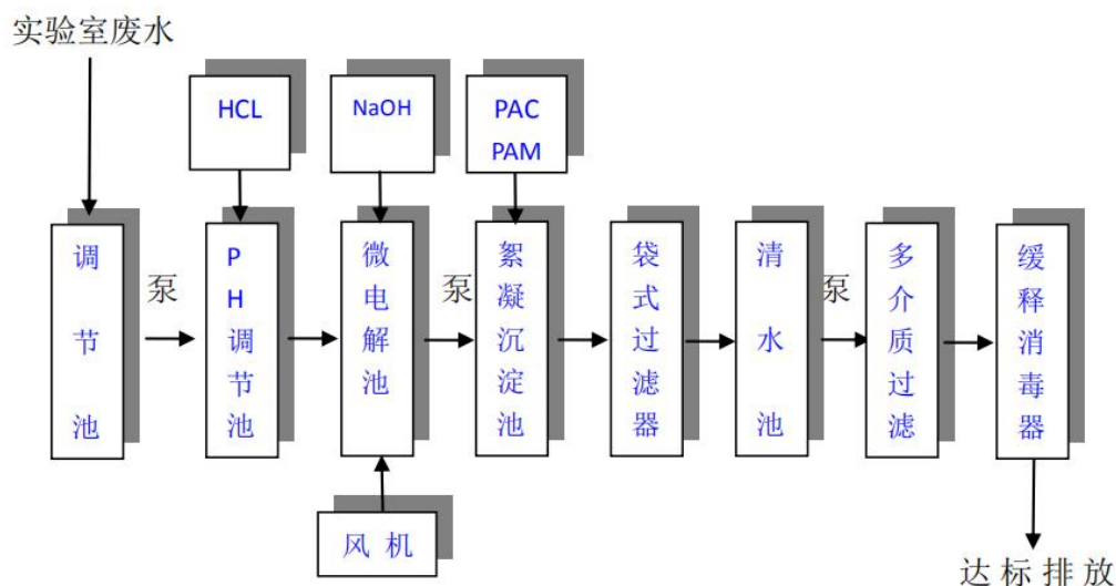
图 4-1 自建一体化污水处理设施污水处理工艺流程
