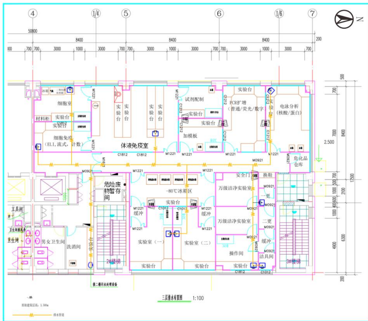
附图 4 项目三层实验区排水走向图
