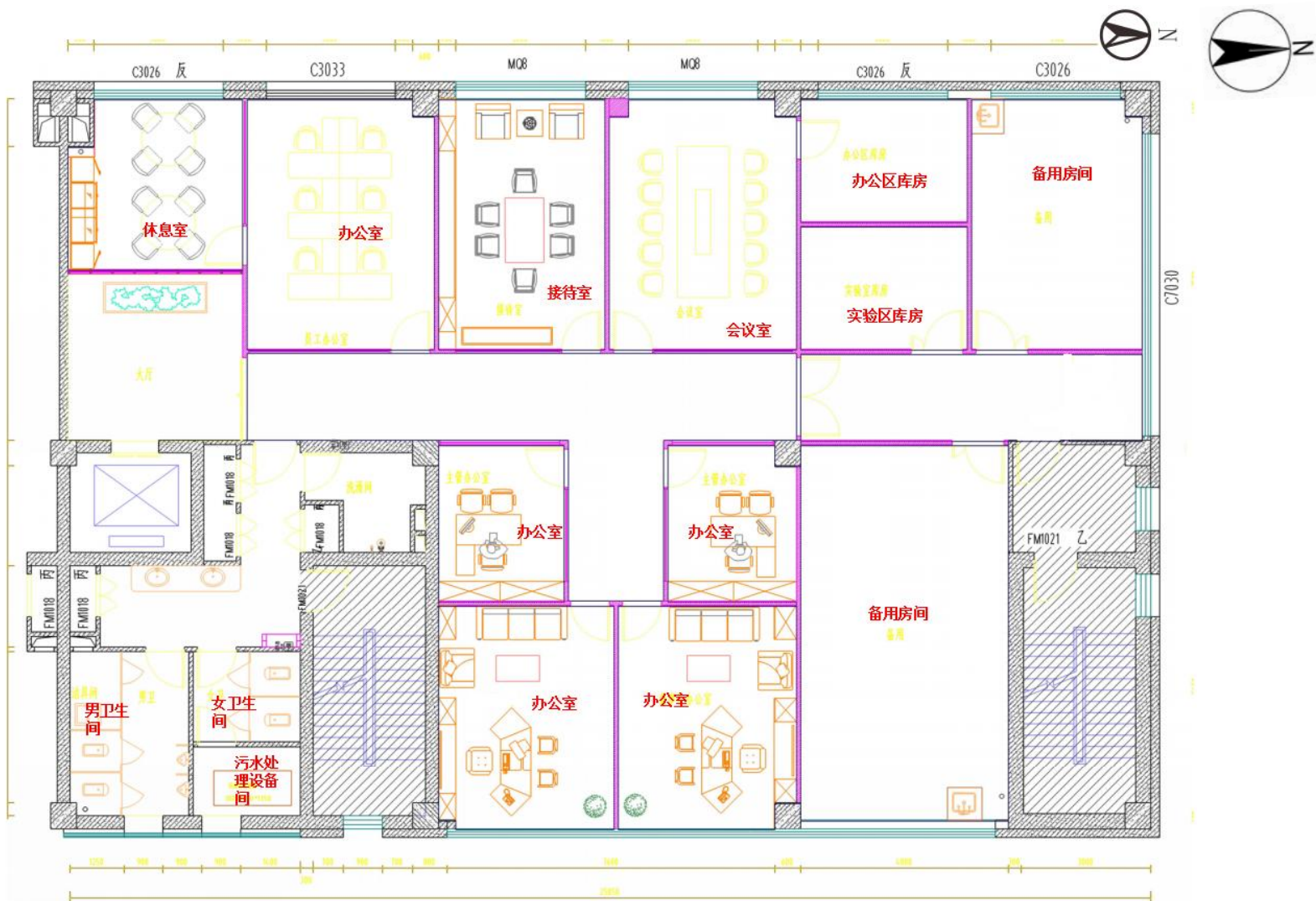
附图 3-1 项目二层办公区平面布置图
