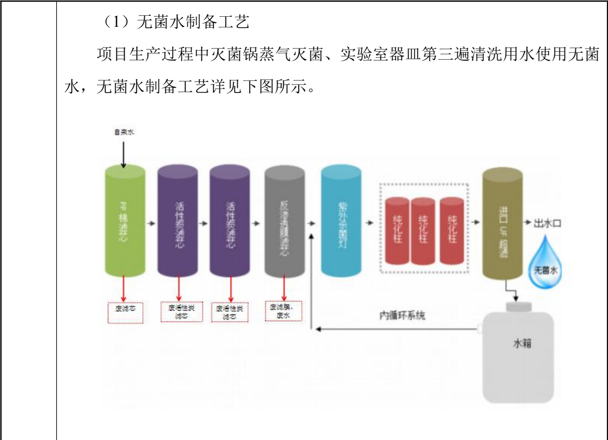
图 2-5 无菌水制备工艺产污环节图示
